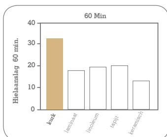
Contact/ Schokdemping
